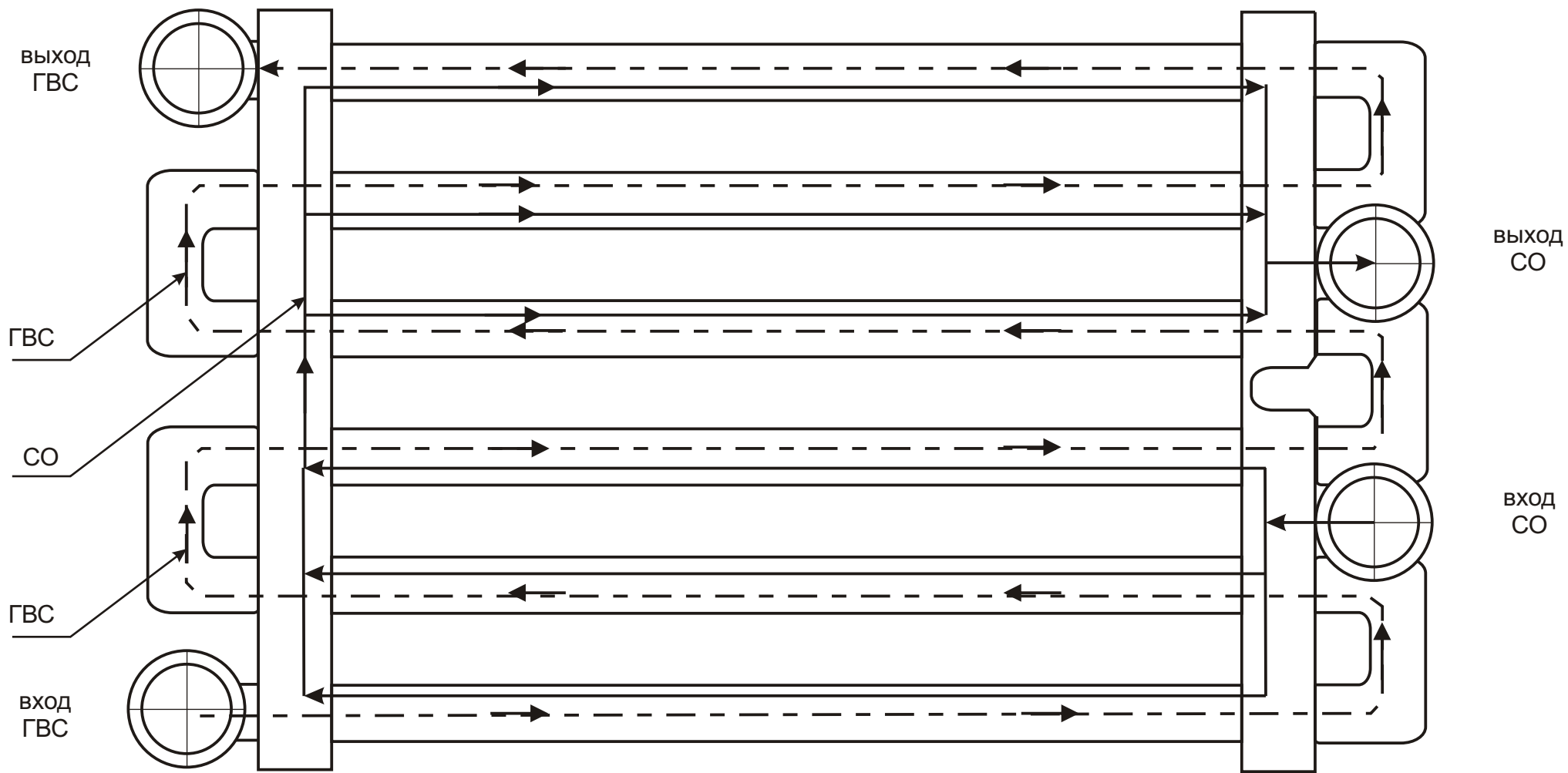
Схема прохождения потоков ГВС и СО в битермальном теплообменнике
